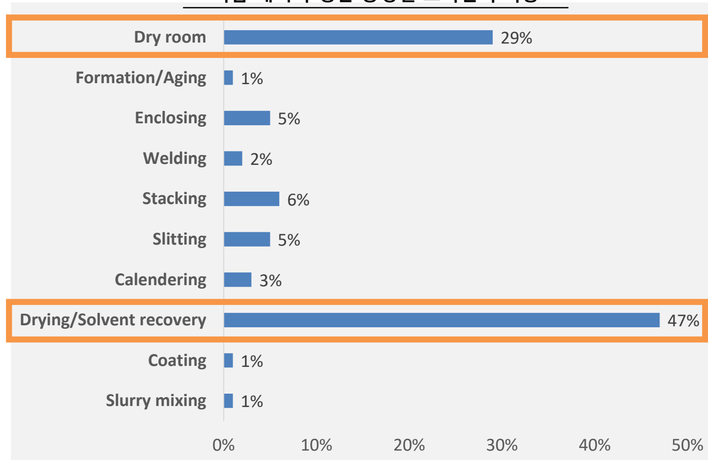
리튬 배터리 생산 공정별 소비전력 비중
