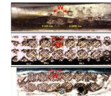
<용접 불량 발생 이미지>
