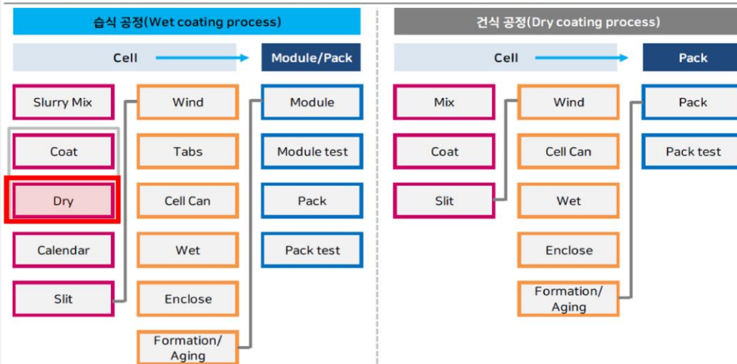
그림 21. 습식 공정(15 가지 공정)과 Tesla의 건식 공정+CTP(Cell to pack) 공정(10 가지 공정) 과정 비교
