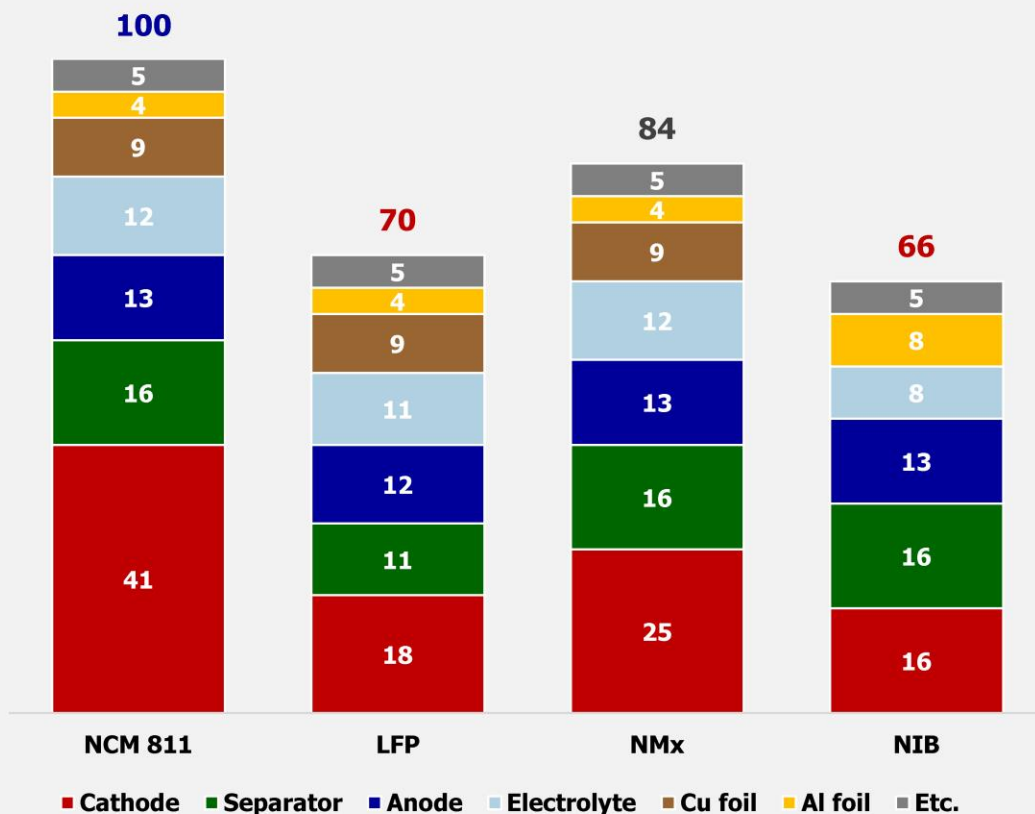
NIB 대비 이차전지 종류별 Cost 가격 구조
