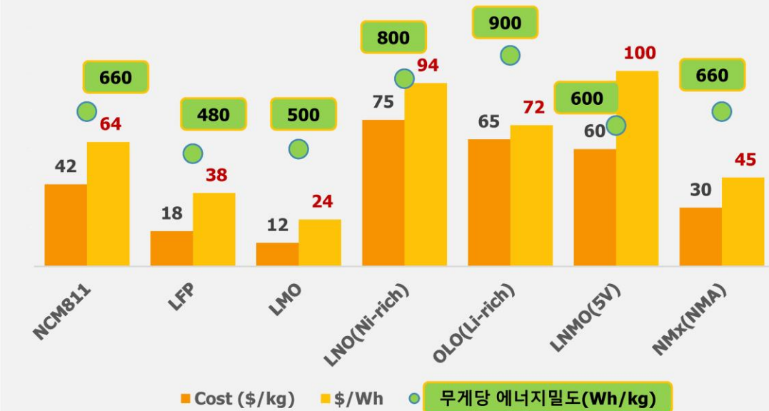
주요 양극재 성능 비교('22년 하반기 Metal 가격 기준)
